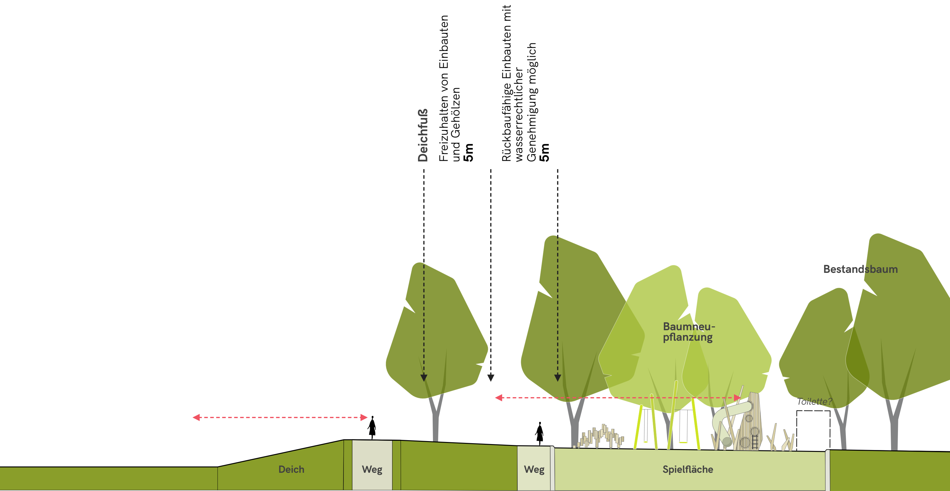
Querschnitt ohne Deicherhöhung M 1:200
