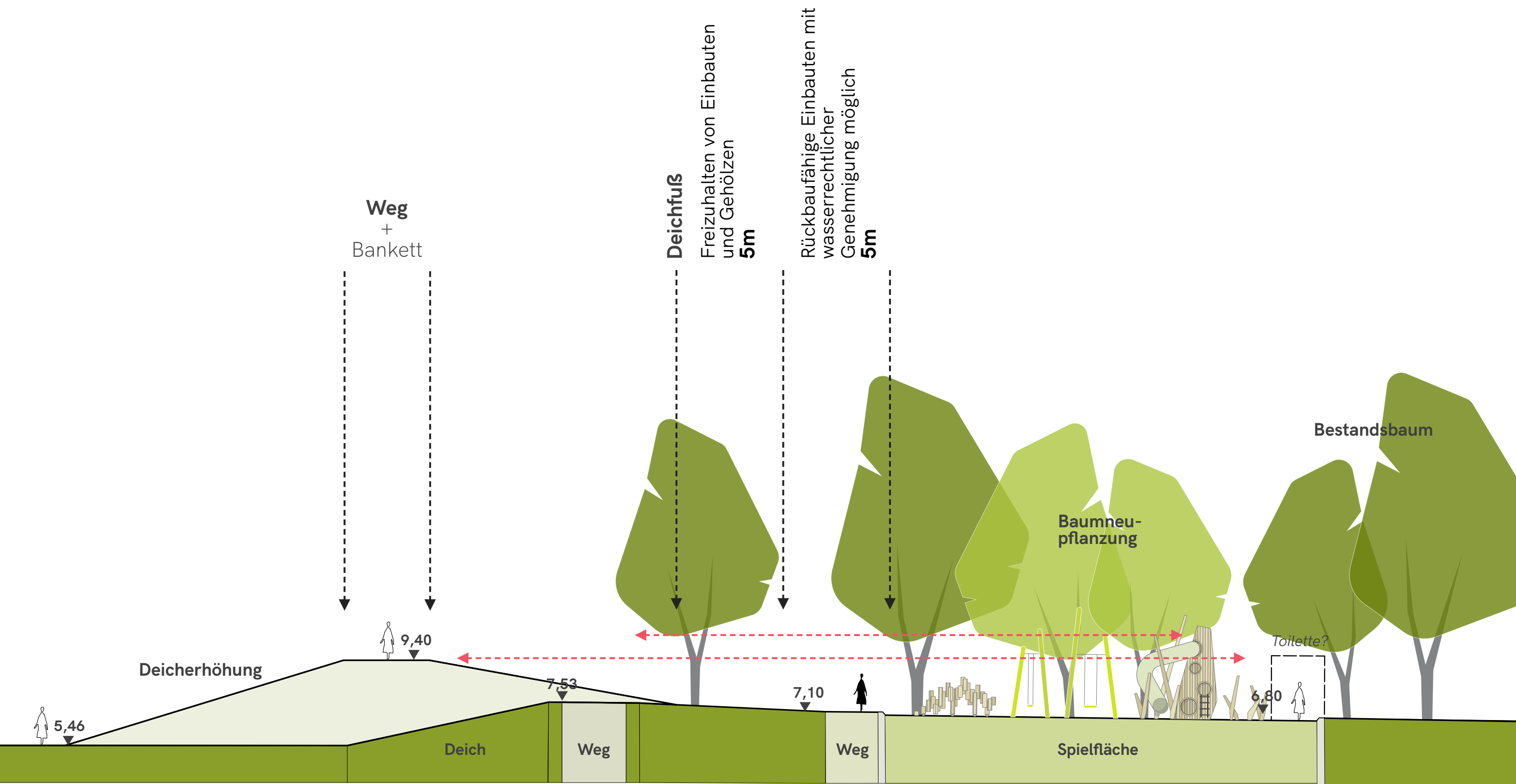
Querschnitt mit Deicherhöhung M 1:200
